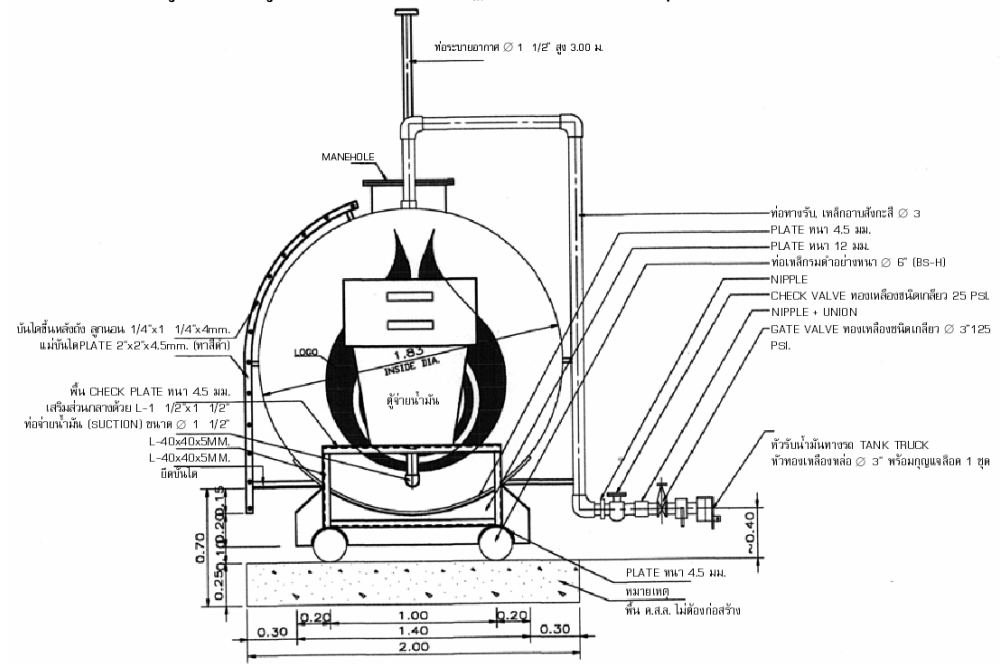
รูปที่ 4-6 รูปด้านหน้าถึงน้ำมันฐานสกีขนาดบรรจุไม่เกิน 9,600 ลิตร
